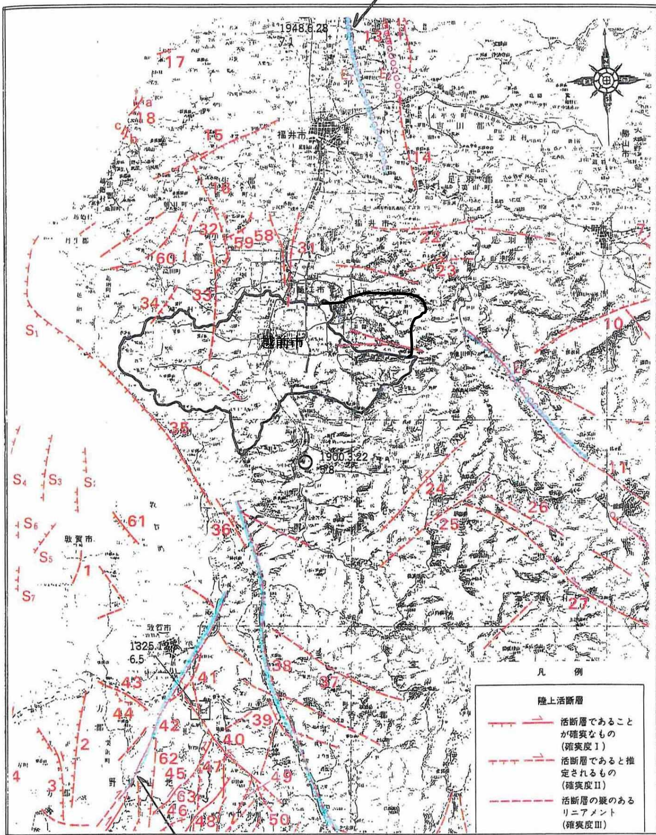
図一3 越前市域周辺の活断層分布図
