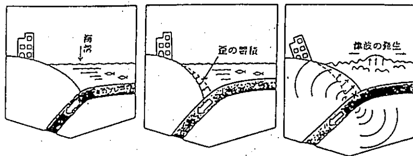
図ー2 海溝型巨大地震発生のメカニズム
