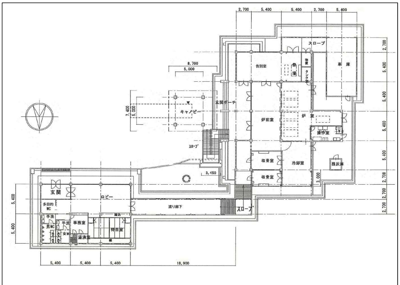
図2 越前市斎場現況平面図
